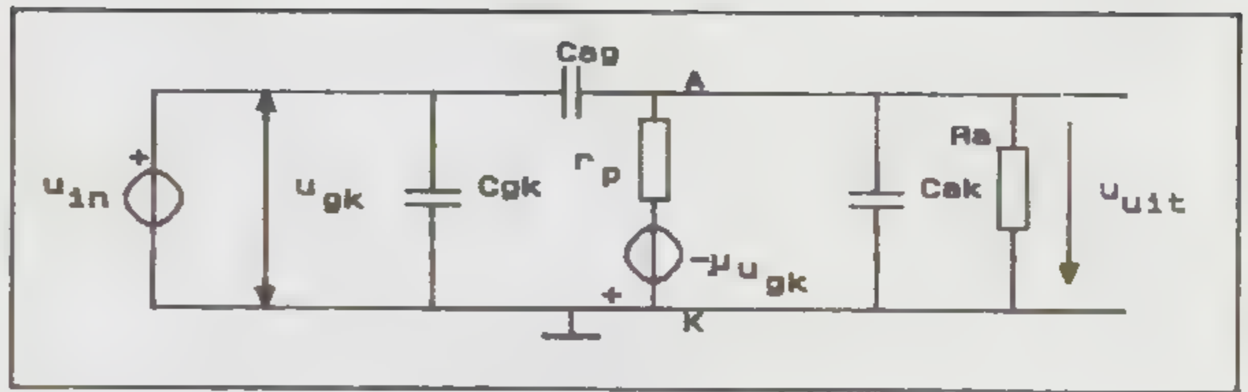
Figuur 15 vervangingschema ECC83
